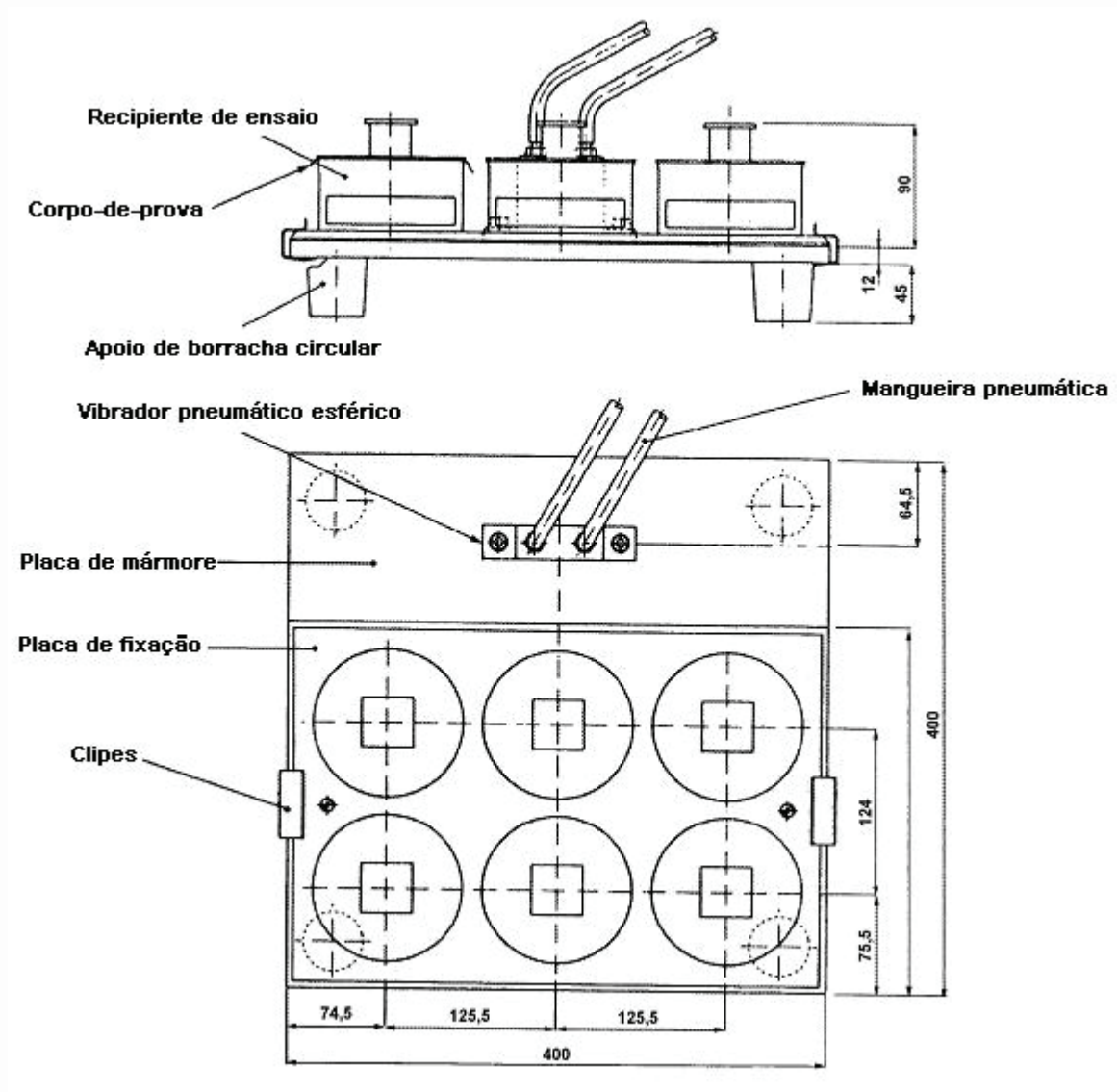
Figura A.1 — Equipamento de ensaio para determinação da penetração bacteriológica a seco
